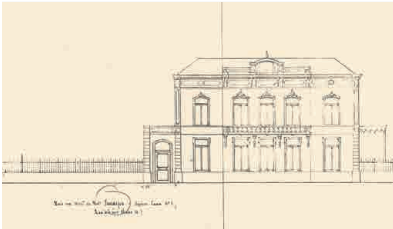
Bouwtekening van de Residentie – gereproduceerd met toestemming van de Gemeente Den Haag.
