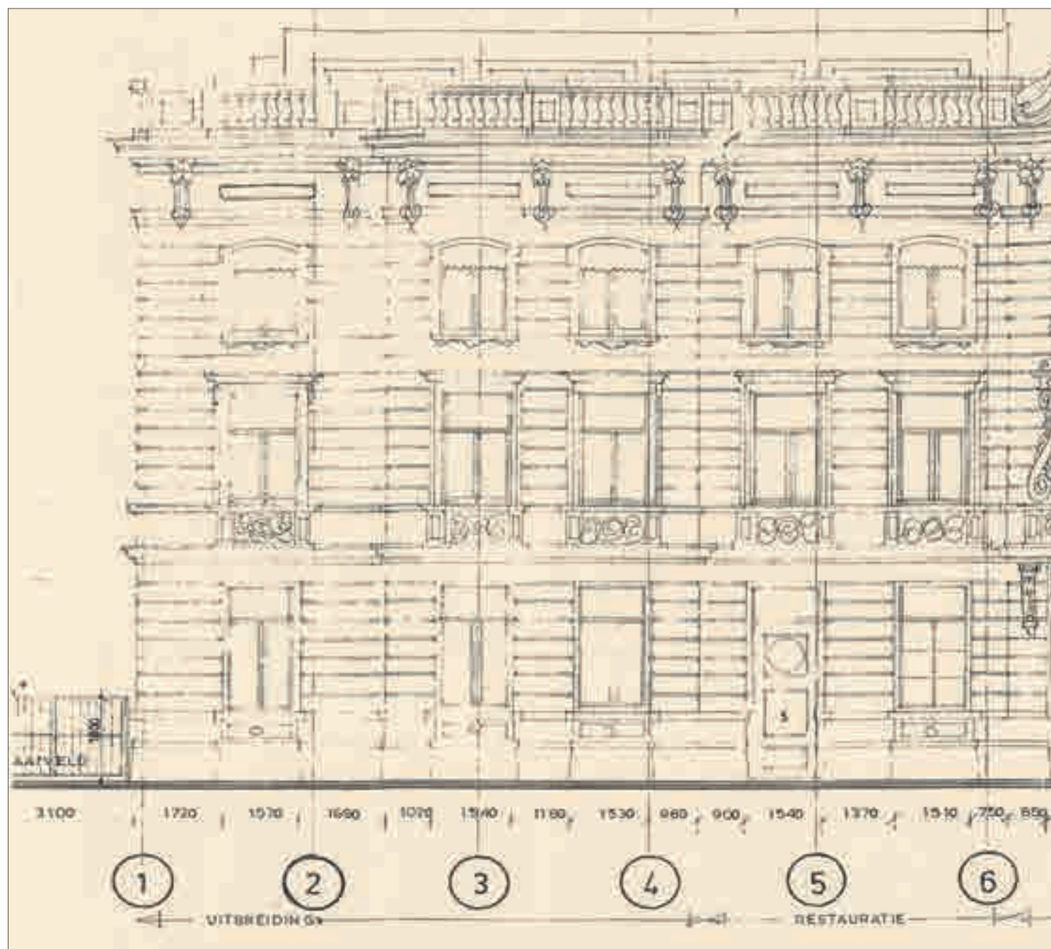
Het gebouw Sophialaan 1-1A. Tekening gereproduceerd met toestemming van de Gemeente Den Haag.
